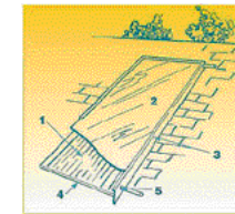
Vue en coupe des éléments d'un capteur plat vitré 1. Absorbant métallique 2. Vitrage 3. Bâti 4. Isolant 5. Entrée du fluide caloporteur
